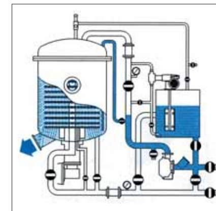
3. LAVAGGIO/ Washing
