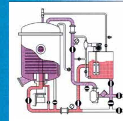
1. FORMAZIONE DEL PANNELLO DA FILTRARE / Unfiltered cake
