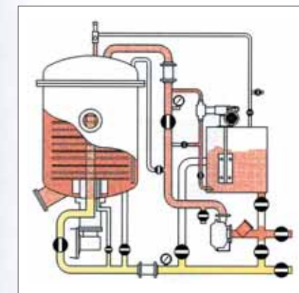
2. FILTRAZIONE/ Filter
