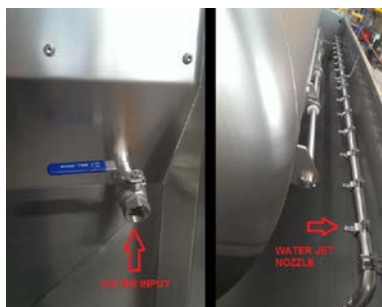
Impianto di lavaggio esterno del tank. Washing system for external tank.
